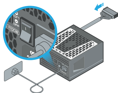
10-poliger Stecker 18-poliger Stecker
